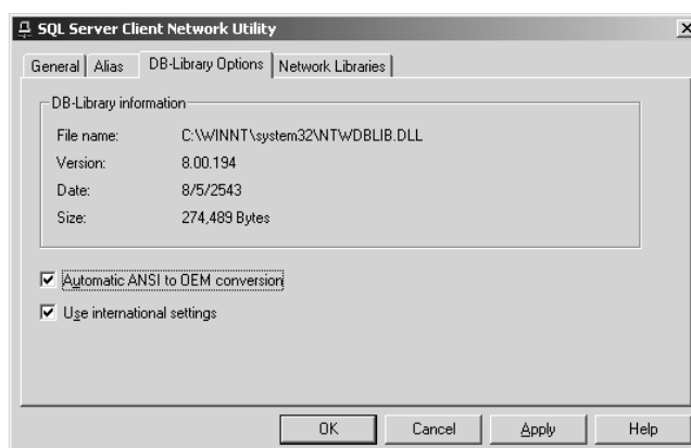
รูปที่ 21 แสดงข้อมูลของไลบรารีของฐานข้อมูล
