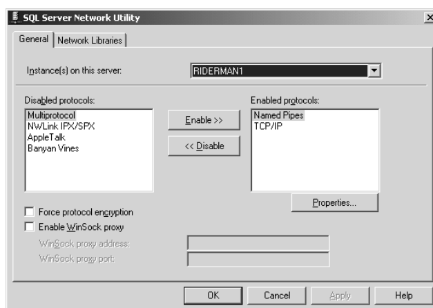
รูปที่ 26 แสดงเครื่องมือกำหนด Network Library ให้กับฝั่ง Server
