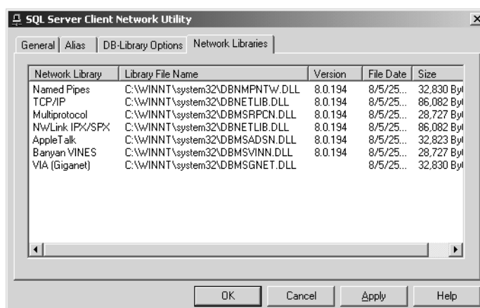
รูปที่ 22 แสดงข้อมูลไลบรารีของเน็ตเวิร์กที่ระบบใช้อยู่
