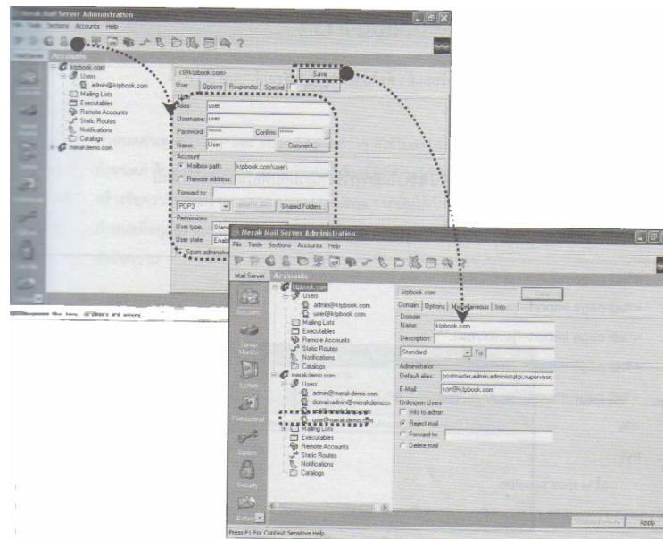
รูปที่ 33 แสดงการเพิ่มผู้ใช้งาน
