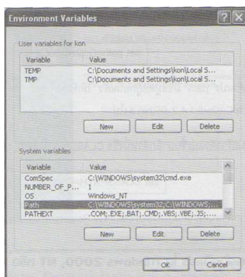
รูปที่ 6 แสดงหน้าต่าง Environment Variable
