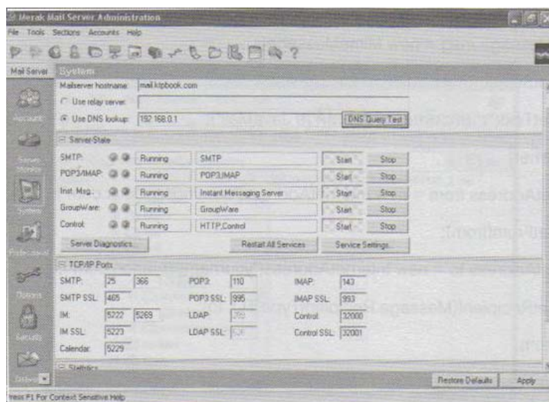
รูปที่ 34 แสดงสถานะต่างๆ ของ service ใน Mail Server
